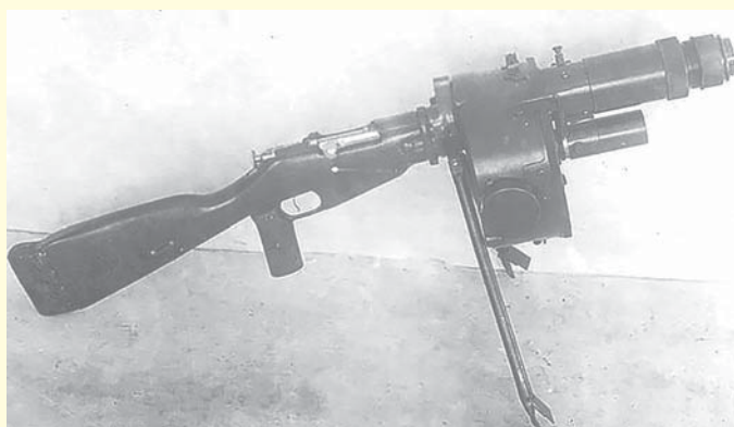
44,15-мм самозарядный гранатомёт конструкции Кулакова
