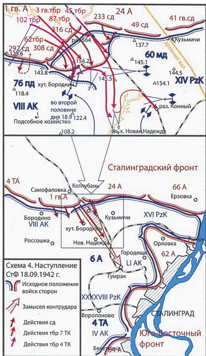
Наступление Сталинградского фронта 18 сентября (отмечены позиции 49-й СД). Карта из книги А.В. Исаева, посвященной Сталинграду
